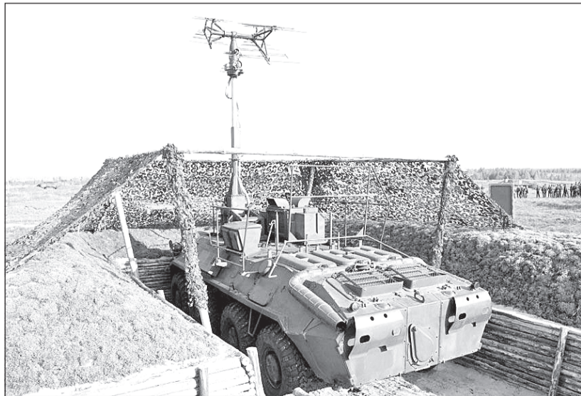
Станция за смущаване на радиовзриватели на артилерийски боеприпаси СПР-2
