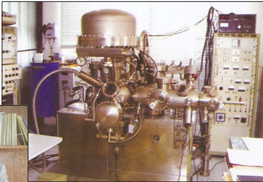
Фотоелектронен спектрометър в института
