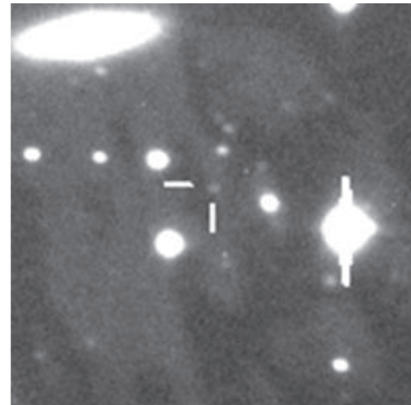
На лявата фигура е показано оригиналното наблюдение с телескопа „Sloan“, а отдясно е показана същата площка, наблюдавана с 2м телескоп на Рожен. Местоположението на кафявото джудже върху двете фигури е маркирано с кръгче и черти съответно
