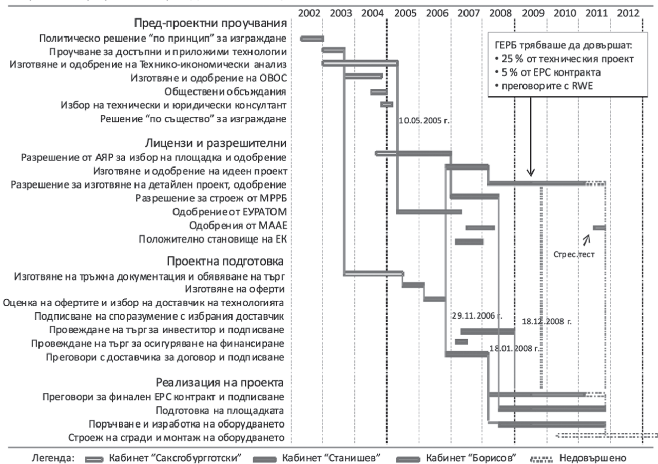
Времеви график за изграждането на АЕЦ „Белене“
